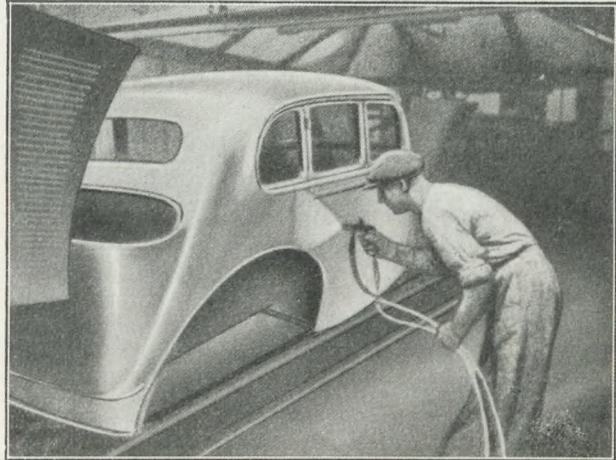
Karosserierne passerer paa Samlerbaandet en Sprøjtekabine, hvor Grundfarven paaføres med Trykluftsprøjte.
