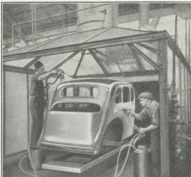
Det sidste Lag Celluloselak paasprøjtes.
